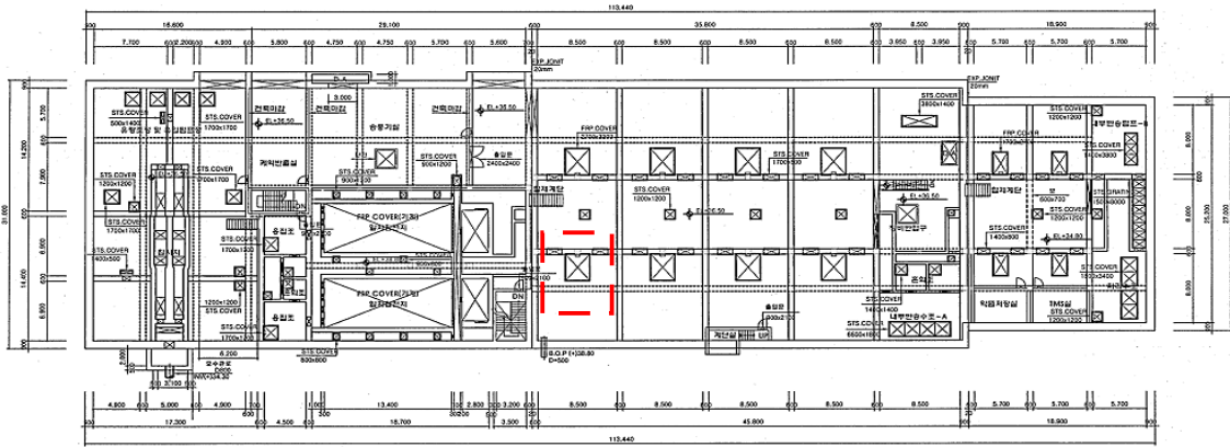
질산화/탈질조 “E” 관련도면
