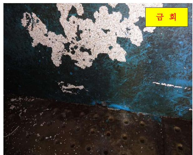
“E” 내부 벽체와 스트레이너 블록 연결부 박락 및 여재 유출 -보수완료-
