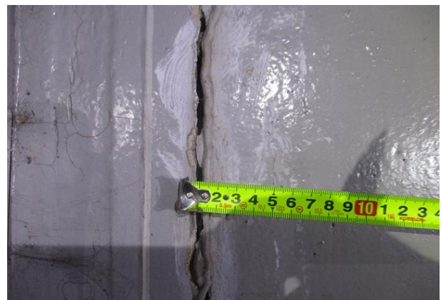
내부 벽체 이음부 이격 ( L=4.0\text{m}\times2\text{EA} , t=0.5\text{cm} )
